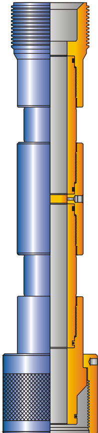
LUBRICATOR RISER
